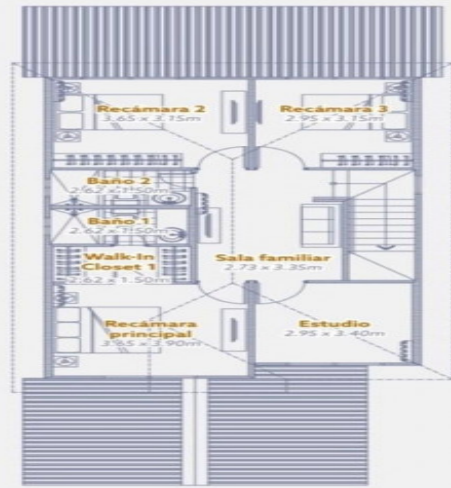
PLANTA ALTA
