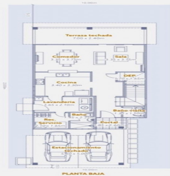
PLANTA BAJA
